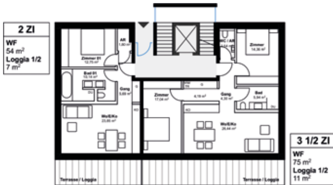
Grundrissvariante 3
