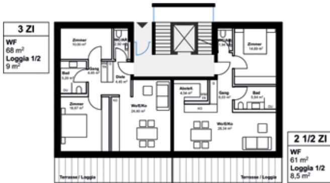
Grundrissvariante 1
